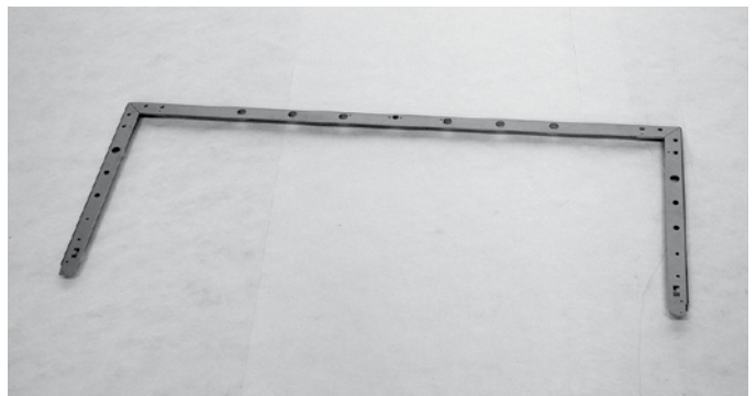
Verstärkungsprofil Stiffening section Profil de renforcement Verstevigingsprofiel
