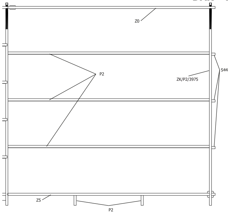
plaatsing van de staalplaten (vooraanzicht) - pose du toit en tôle (vue de face)
