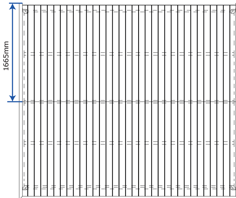
DAK - TOITURE
