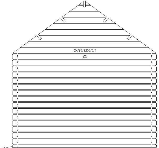
DAK - TOITURE
